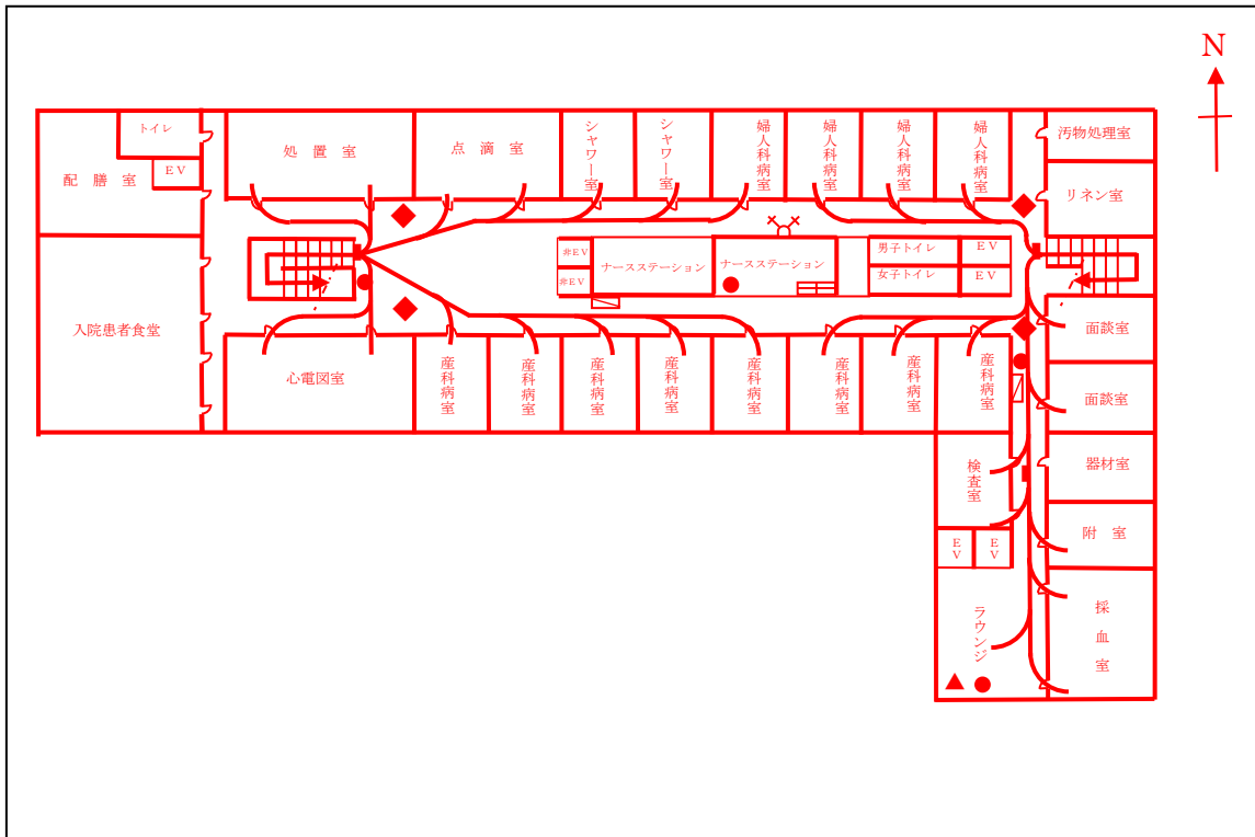
1 1階平面図
