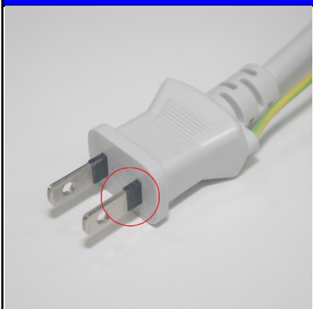
トラッキング現象防止プラグ
